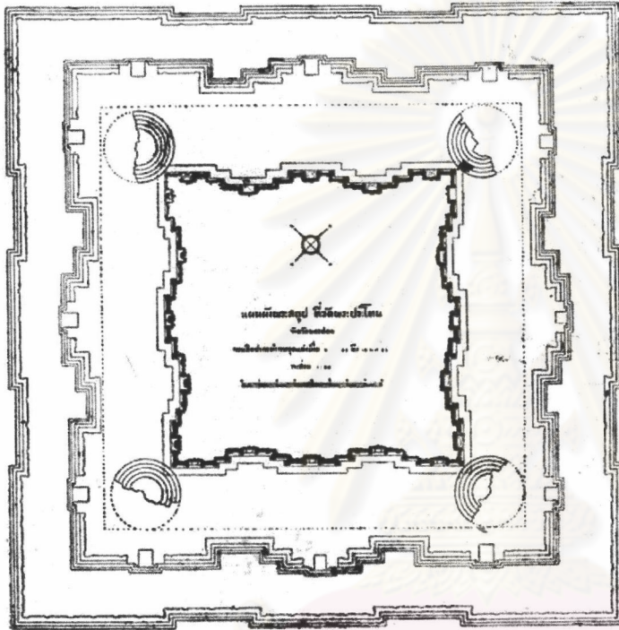
แผนผังที่ 2-1 เจดีย์จุลประโทน วัดพระประโทน นครปฐม มีอายุระหว่างพุทธศตวรรษที่ 10-14 ได้ปรักหักพังเหลือแต่เฉพาะส่วนฐาน ลักษณะเป็นฐานสี่เหลี่ยมย่อมุม และทำเป็นช่องประดับภาพชดากโดยรอบ ตั้งซ้อนบนฐานสี่เหลี่ยมสองชั้น ใช้เป็นลานประทักษิณ ที่ลานมีบันไดยื่นออกไปทั้งสี่ทิศ เป็นอัญจันทร์รอบทุกด้าน 10
