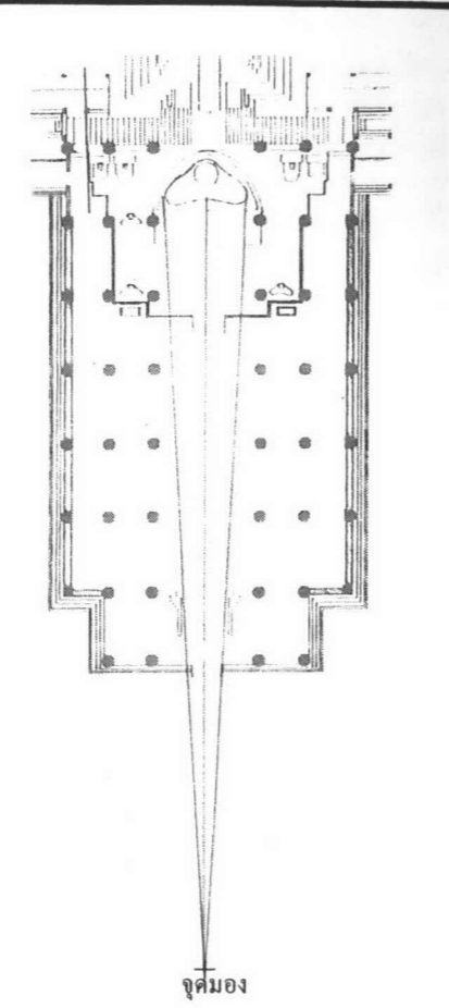
ผังวิหารวัดพระศรีรัตนมหาธาตุ เมืองศรีสัชนาลัย
