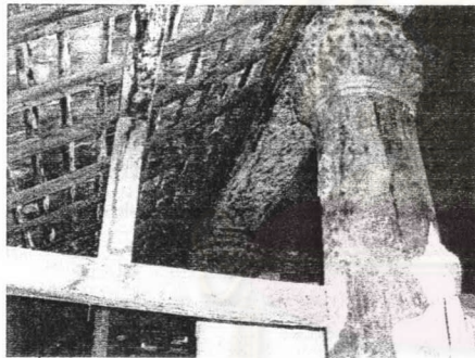
รูปที่ 5.2.51 ภาพแสดงโครงสร้างในวิหารวัดวังทอง มีสะพานรับแผงคอสองอยู่เหนือหัวเสา
