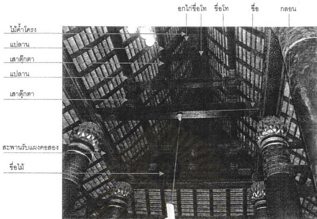
รูปที่ 5.2.50 ภาพแสดงโครงสร้างหลังคาภายในวิหารวัดราชบูรณะ
