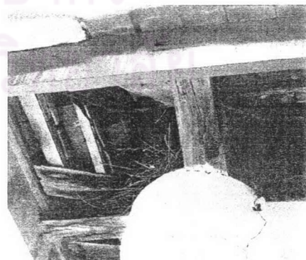
รูปที่ 5.2.54 ภาพแสดงปลายเด้าที่มีเดือยยื่นมารับเชิงกลอน ที่วิหารวัดวังทอง
