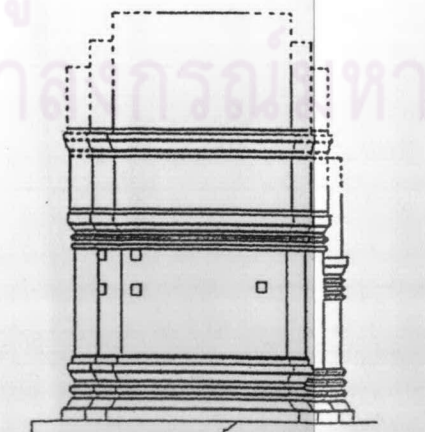
รูปด้านข้างคันทอกรีตวัดสระไ้
