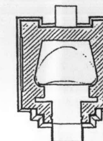
ผังคันทอกรีตส่วนพระอุโบสถวัดกุฎีราย เมืองศรีสะเกษ
