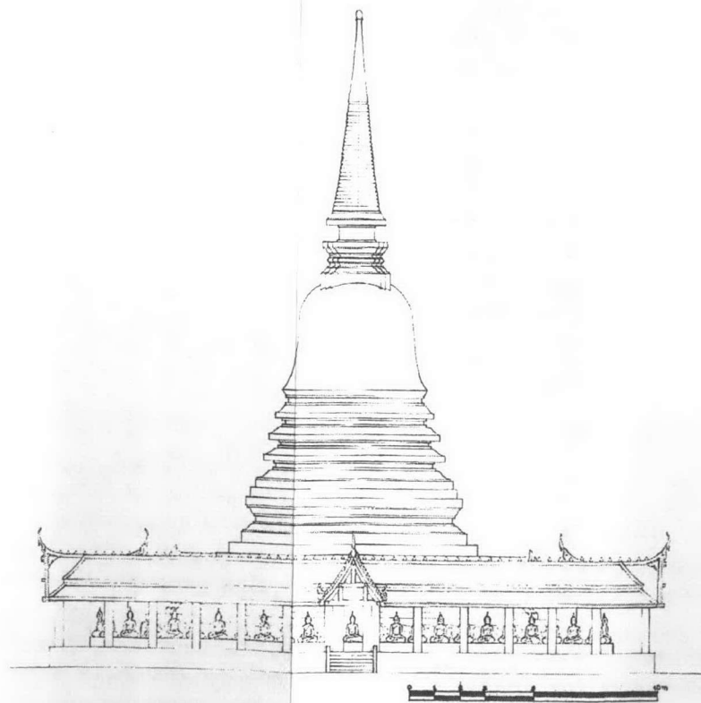
ภาพลายเส้นที่ 5.2.10 รูปด้านของพระเจดีย์ช้างล้อมในสมัยอยุธยา
