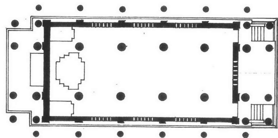
ภาพถ่ายเส้นที่ 5.2.30 ผังพระอุโบสถสมัยสุโขทัยแบบที่ 2
