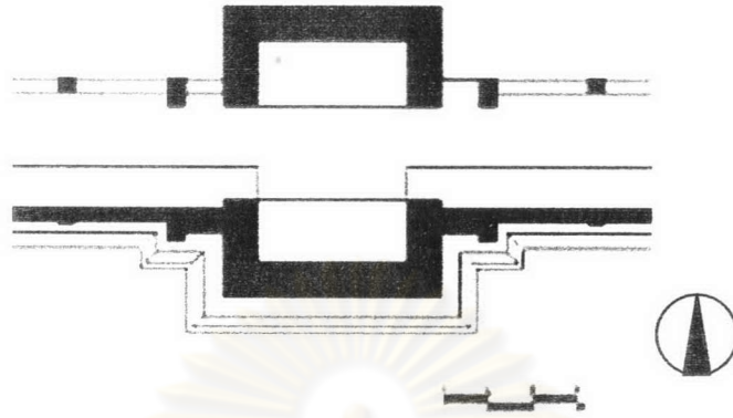
ภาพลายเส้นที่ 5.2.49 ผังพื้นพระระเบียงคด และ ชุ่มพระ
