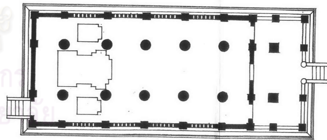
ภาพถ่ายเส้นที่ 5.2.26 ผังพระอุโบสถสมัยอยุธยา
