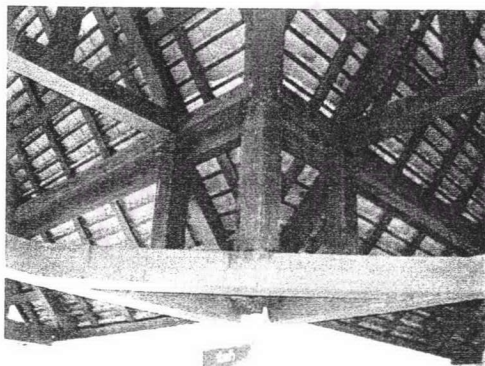
รูปที่ 5.2.91 โครงสร้างหลังคาพระระเบียงคดมีการใช้ข้อฝากกับ ข้อหลักเพื่อรับเสาดั้งที่รับหลังคาชั้นบน
