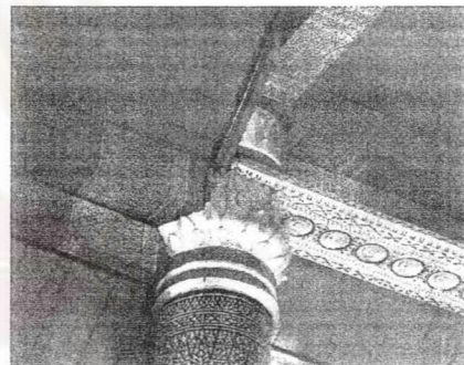
รูปที่ 5.2.52 ภาพแสดงโครงสร้างในวิหารพระพุทธชินราช มีสะพานรับแผงคอสองอยู่เหนือหัวเสา
