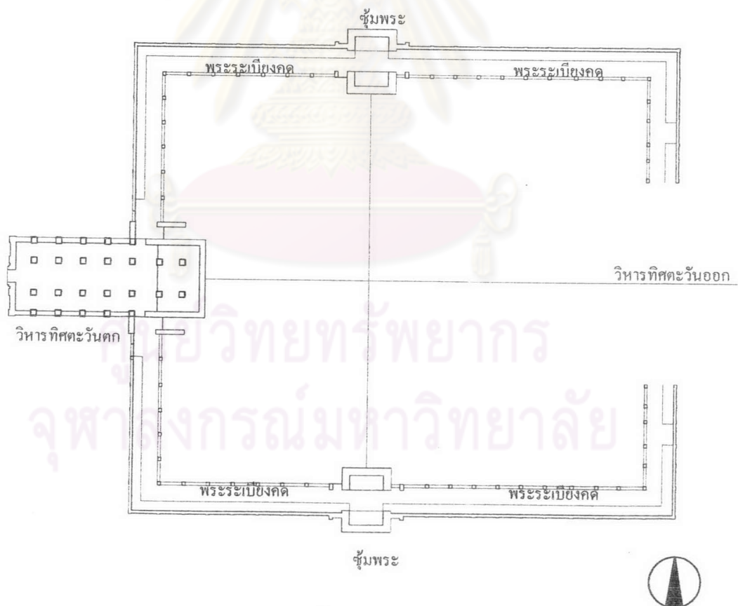
ภาพลายเส้นที่ 5.2.48 ผังพื้นพระระเบียงคด ชุ่มพระ และ พระวิหารทิศตะวันตก
