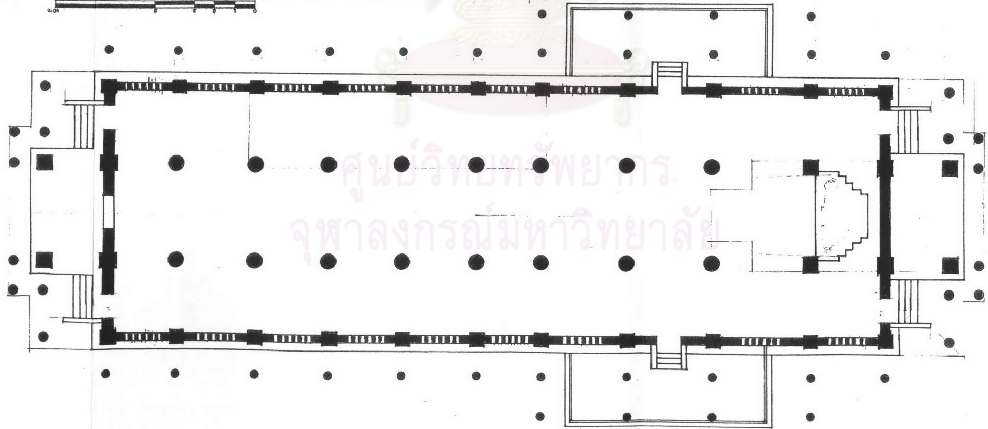
ภาพลายเส้นที่ 5.2.20 ผังพระวิหารวัดอรุณราชวรารามราชวรมหาวิหาร กรุงเทพมหานคร
