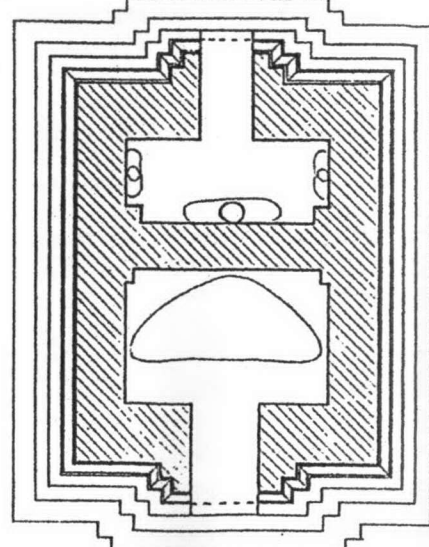
ผังคันทอกรีตวัดพญาดำ เมืองศรีสะเกษ
