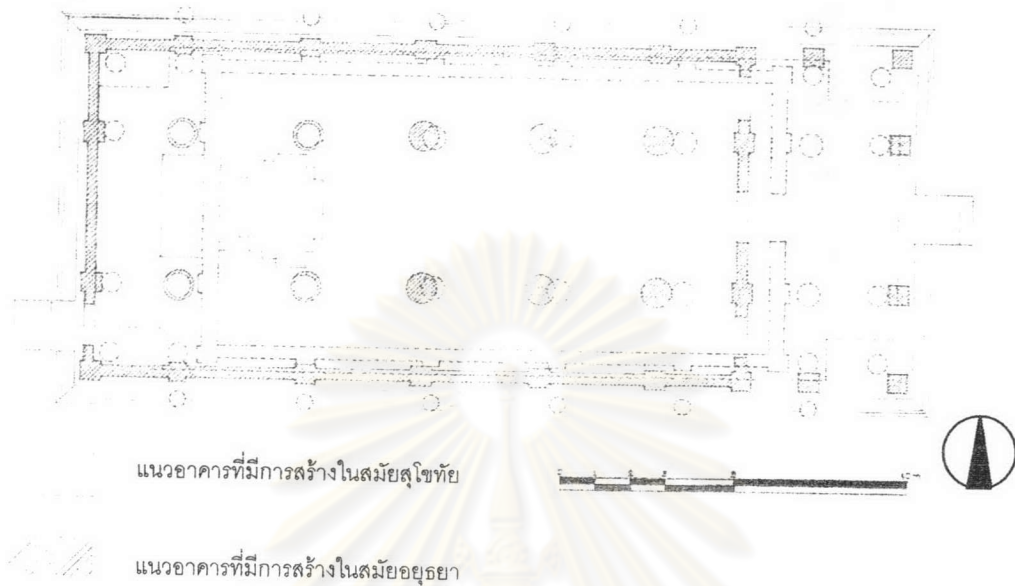
ภาพลายเส้นที่ 5.2.26 ผังแสดงแนวอาคารของพระอุโบสถในแต่ละสมัย
