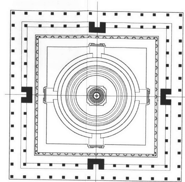
ภาพลายเส้นที่ 5.2.8 ผังพื้นของพระเจดีย์ช้างล้อมในสมัยอยุธยา
