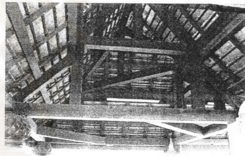
รูปที่ 5.2.90 โครงสร้างหลังคาของพระวิหารมีการยก ชั้นลดของหลังคาเป็นสองชั้น
