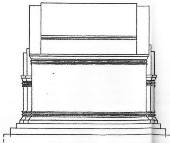
รูปด้านข้างคันทอกรีตวัดพญาดำ
