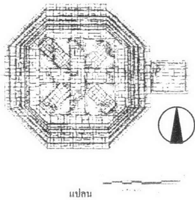
แปลน
