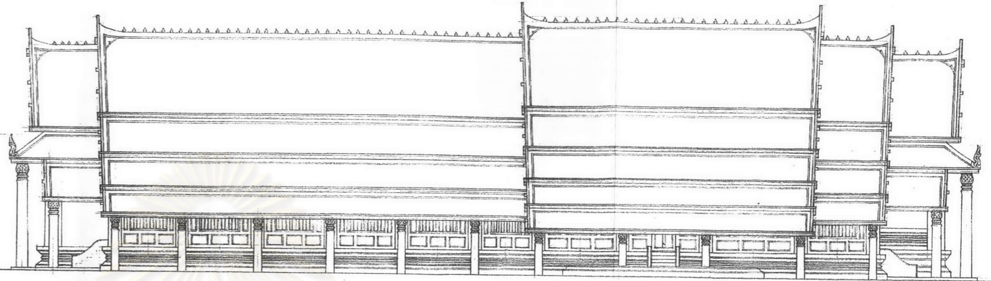
ภาพลายเส้นที่ 5.2.23 รูปด้านข้างพระวิหารวัดอรัญญิก เมืองพิษณุโลกในสมัยสุโขทัย
