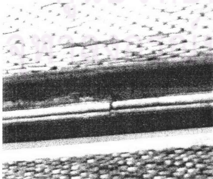
รูปที่ 5.2.53 ภาพแสดงปลายเด้าที่มีเดือยยื่นมารับเชิงกลอน ที่วิหารวัดราชบูรณะ
