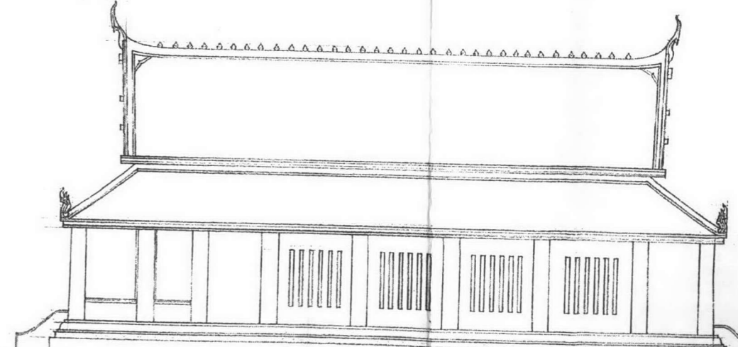
ภาพถ่ายเส้นที่ 5.2.38 รูปด้านข้างพระอุโบสถสมัยอยุธยา
