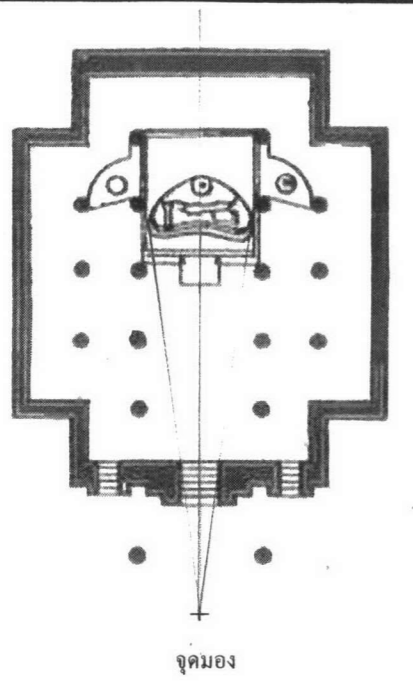
ผังวิหารวัดเจติยคีรีห้อย เมืองสุโขทัย
