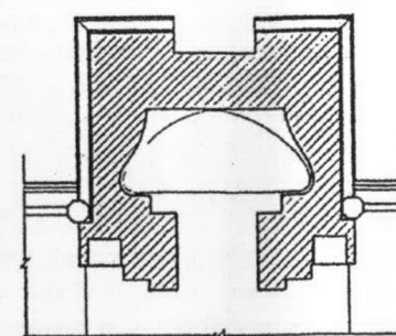
ผังคันทอกรีตวัดชมชื่น เมืองศรีสะเกษ
