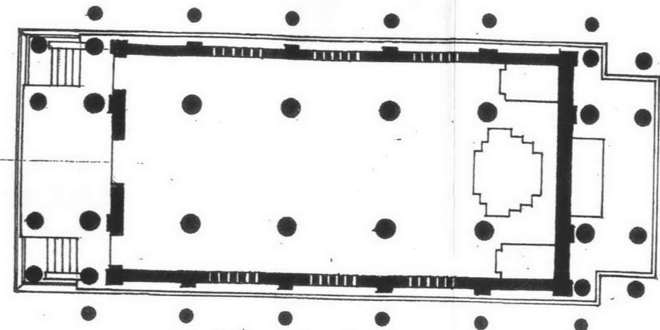
ภาพถ่ายเส้นที่ 5.2.33 ผังพระอุโบสถสมัยสุโขทัยแบบที่ 3
