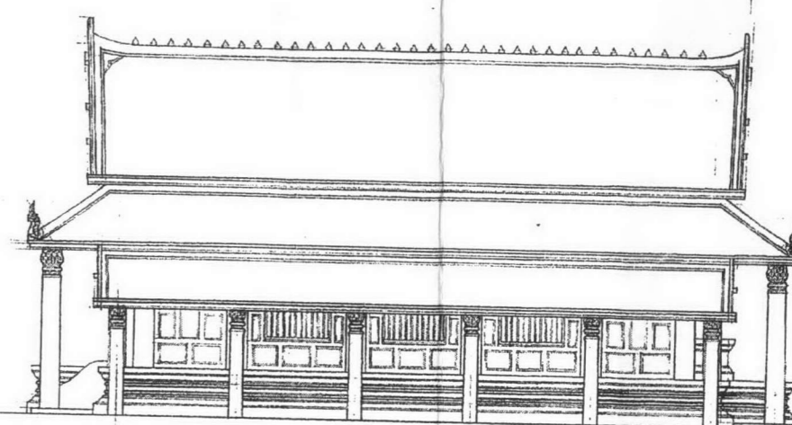
ภาพถ่ายเส้นที่ 5.2.35 รูปด้านข้างพระอุโบสถสมัยสุโขทัยแบบที่ 3
