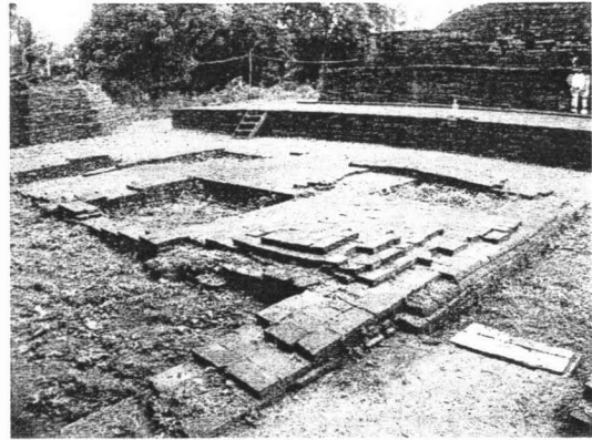
รูปที่ 5.2.83 แนวการก่ออิฐฐานรากของพระวิหาร
