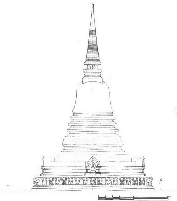
ภาพลายเส้นที่ 5.2.9 รูปด้านของพระเจดีย์ช้างล้อมในสมัยสุโขทัย
