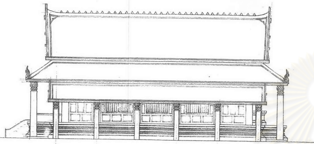
ภาพถ่ายเส้นที่ 5.2.29 รูปด้านข้างพระอุโบสถสมัยสุโขทัยแบบที่ 1
