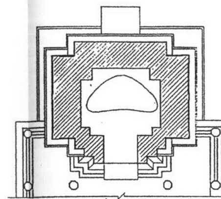
ผังคันทอกรีตส่วนพระวิหารวัดกุฎีราย เมืองศรีสะเกษ
