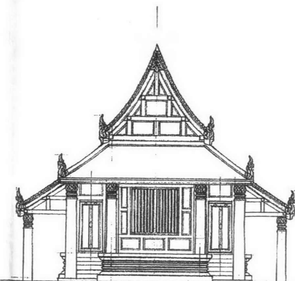
ภาพถ่ายเส้นที่ 5.2.31 รูปด้านหน้าพระอุโบสถสมัยสุโขทัยแบบที่ 2
