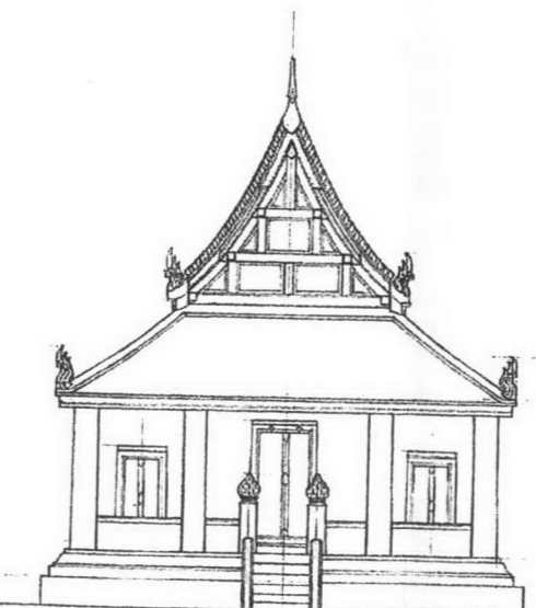
ภาพถ่ายเส้นที่ 5.2.37 รูปด้านหน้าพระอุโบสถสมัยอยุธยา
