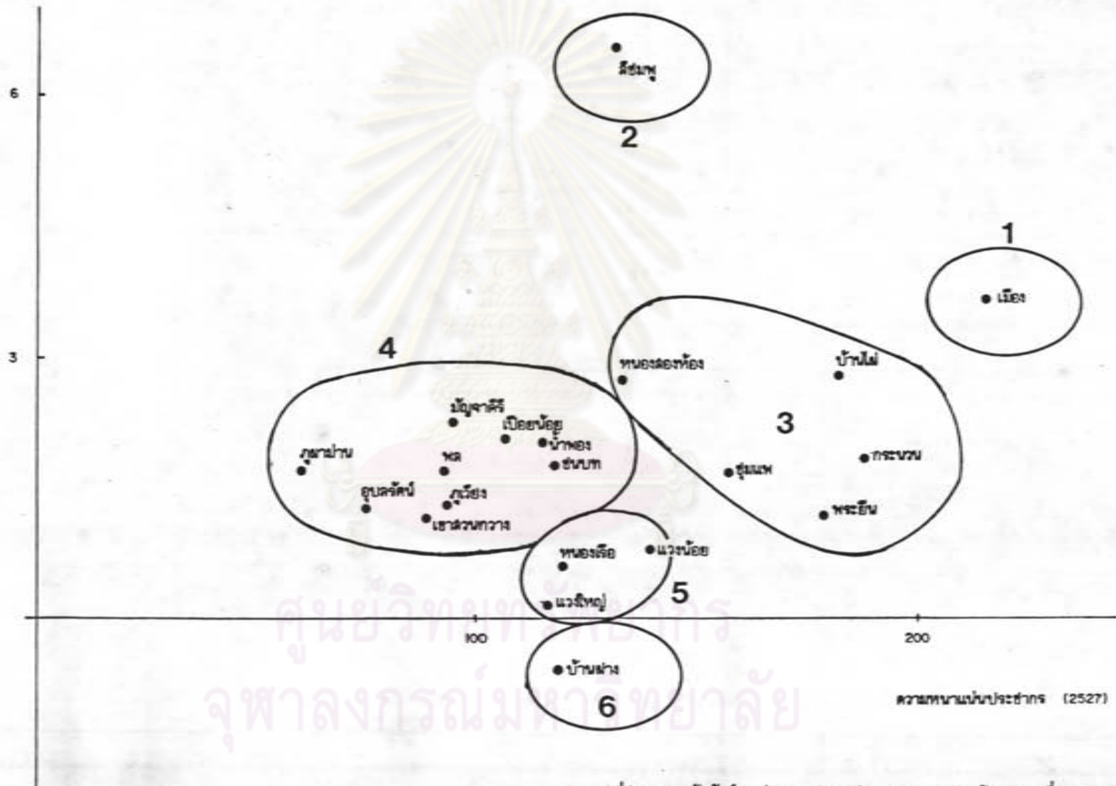
แผนภูมิที่ 4.3 ความสัมพันธ์ระหว่างความหนาแน่นประชากรและอัตราการเปลี่ยนแปลงประชากร
