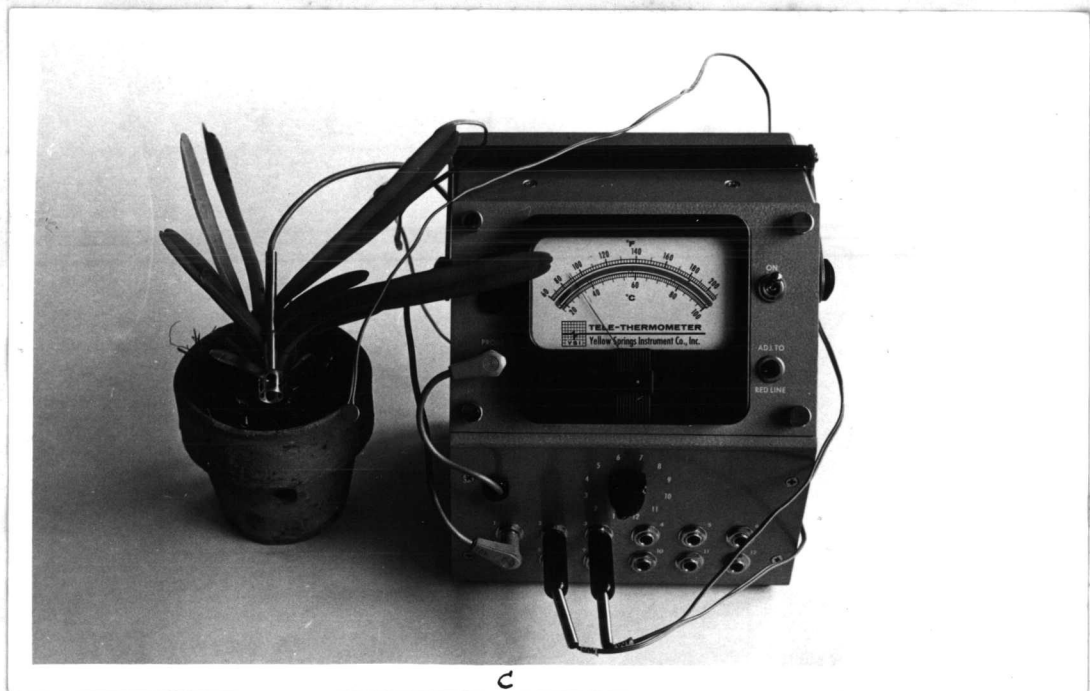
C. เครื่อง Tele - Thermometer ของ Yellow Spring Instrument Co. Inc., model no. ๘๘ TC
