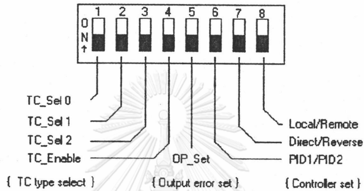
รูปที่ 3.2 แสดงตำแหน่งต่างๆ ของดิฟสวิตช์
