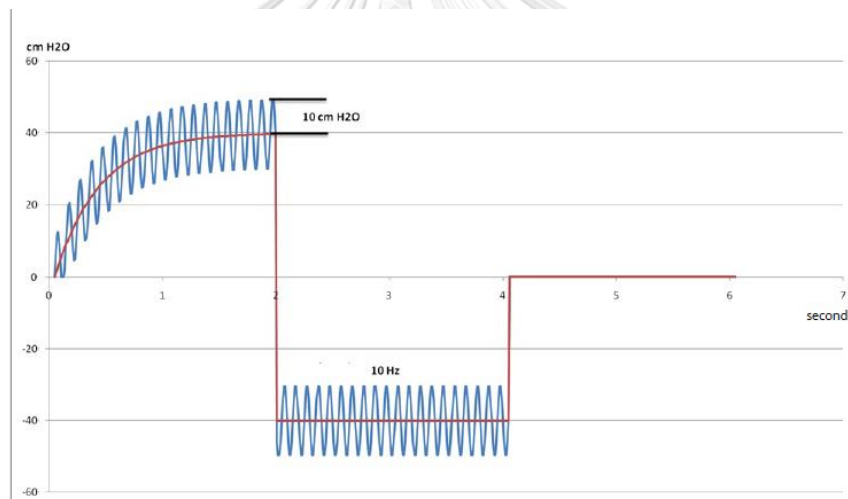
รูปภาพที่ 12 แสดงตัวอย่างการตั้งค่า amplitude และ frequency
