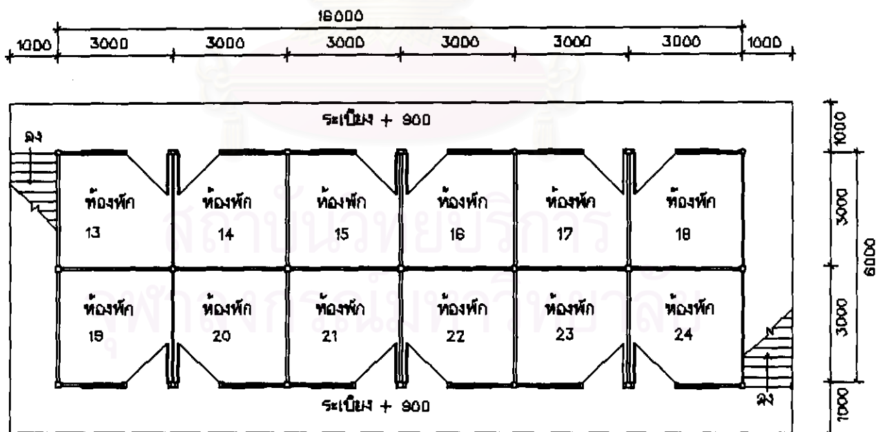
แปลนพื้นที่บน มาตรฐาน 1 : 100
