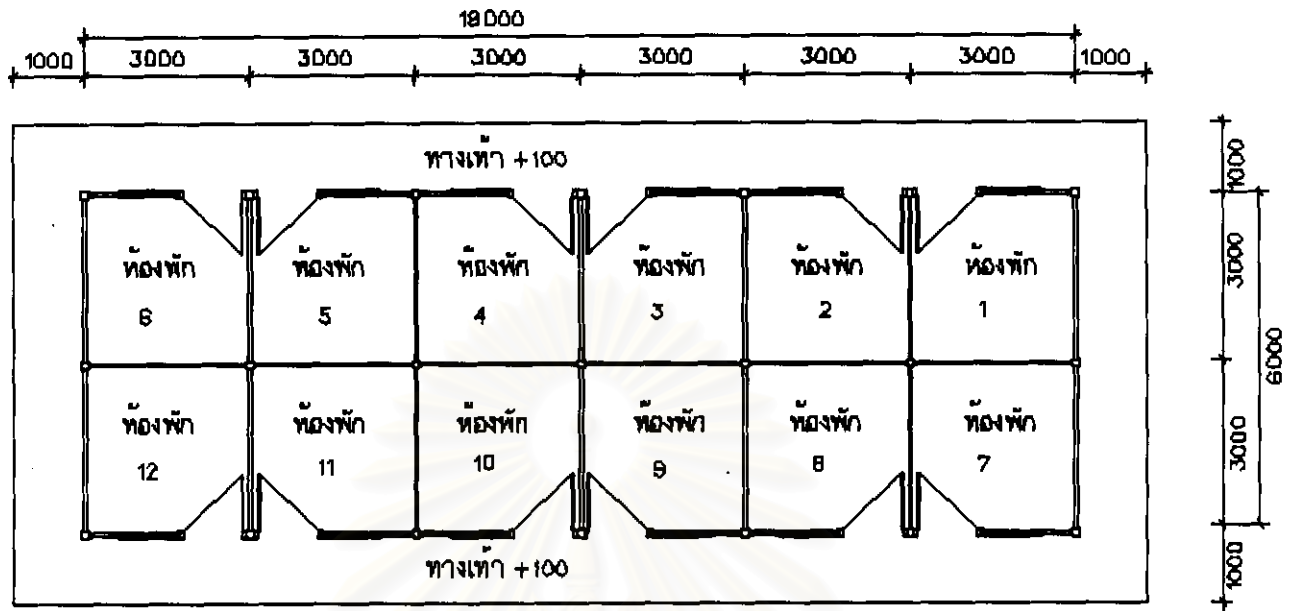
แปลนพื้นที่ชั้นล่าง มาตราส่วน 1 : 100
