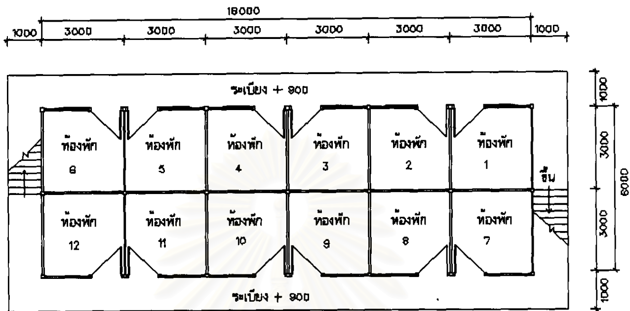
แปลนพื้นที่กลาง มาตรฐาน 1 : 100
