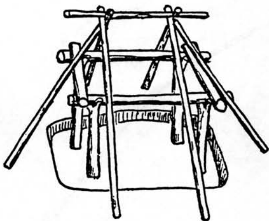
ก. ที่อยู่อาศัยแบบหลุมของโจมนอน โครงสร้างตัวอาคาร ข. ที่อยู่อาศัยแบบหลุมของโจมนอน รูปร่างอาคารที่สร้างขึ้นใหม่
