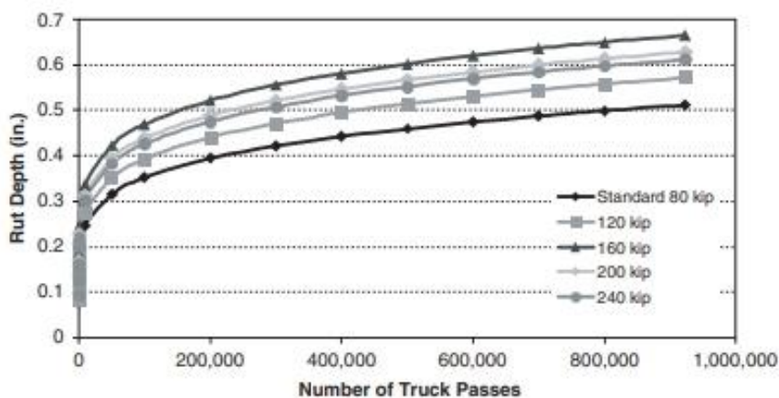
รูปที่ 2 ผลวิเคราะห์กราฟความลึกร่องล้อ สำหรับรถบรรทุกที่ศึกษา
