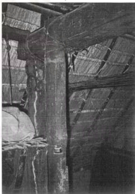
รูปที่ 47 วิธีการมัดด้วยหวายแบบทั่วไป ของเสาไม้ไผ่กะบะเตาไฟ และซื่อ
