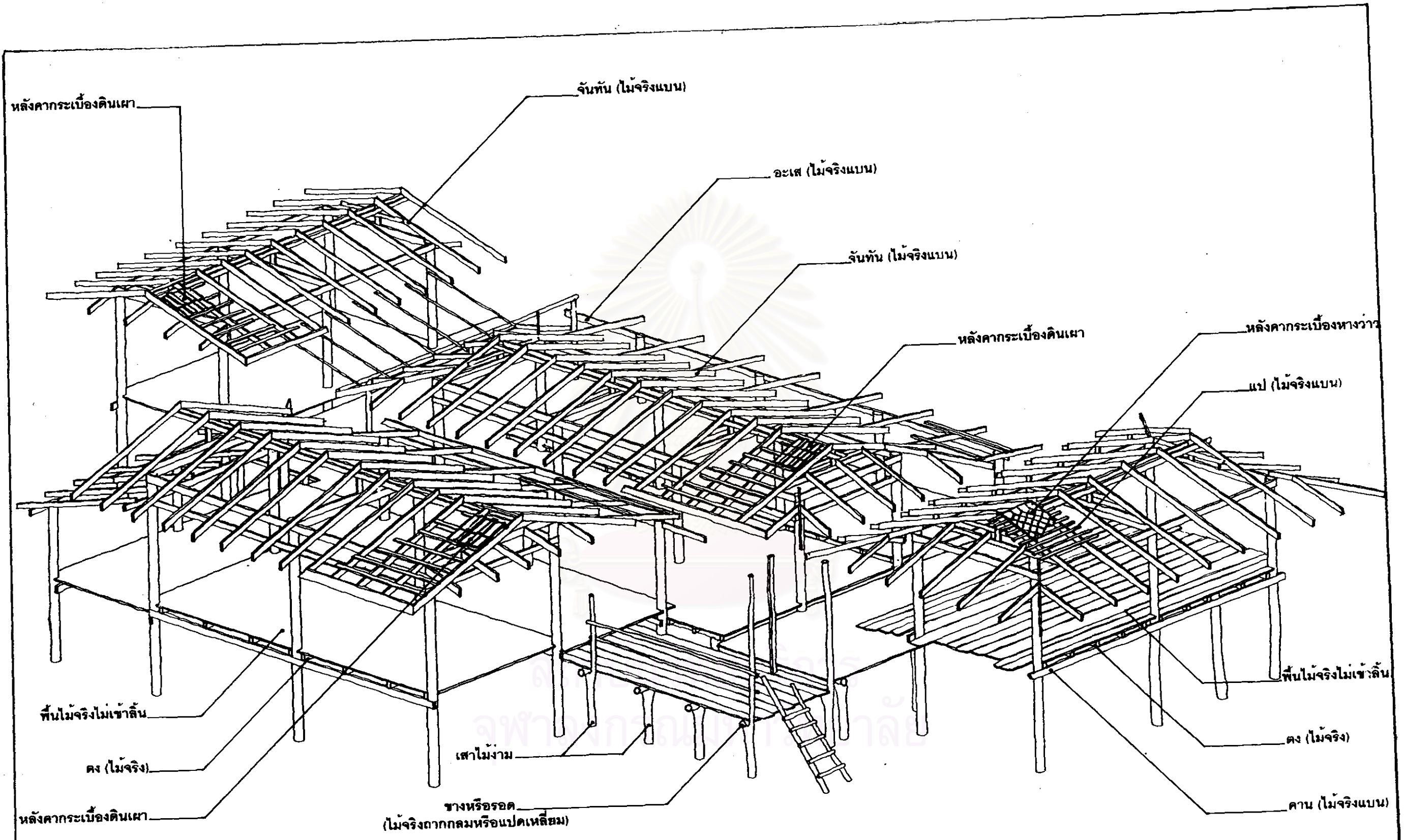
โครงสร้างเรือนนางเขียด เรืองย้อย
