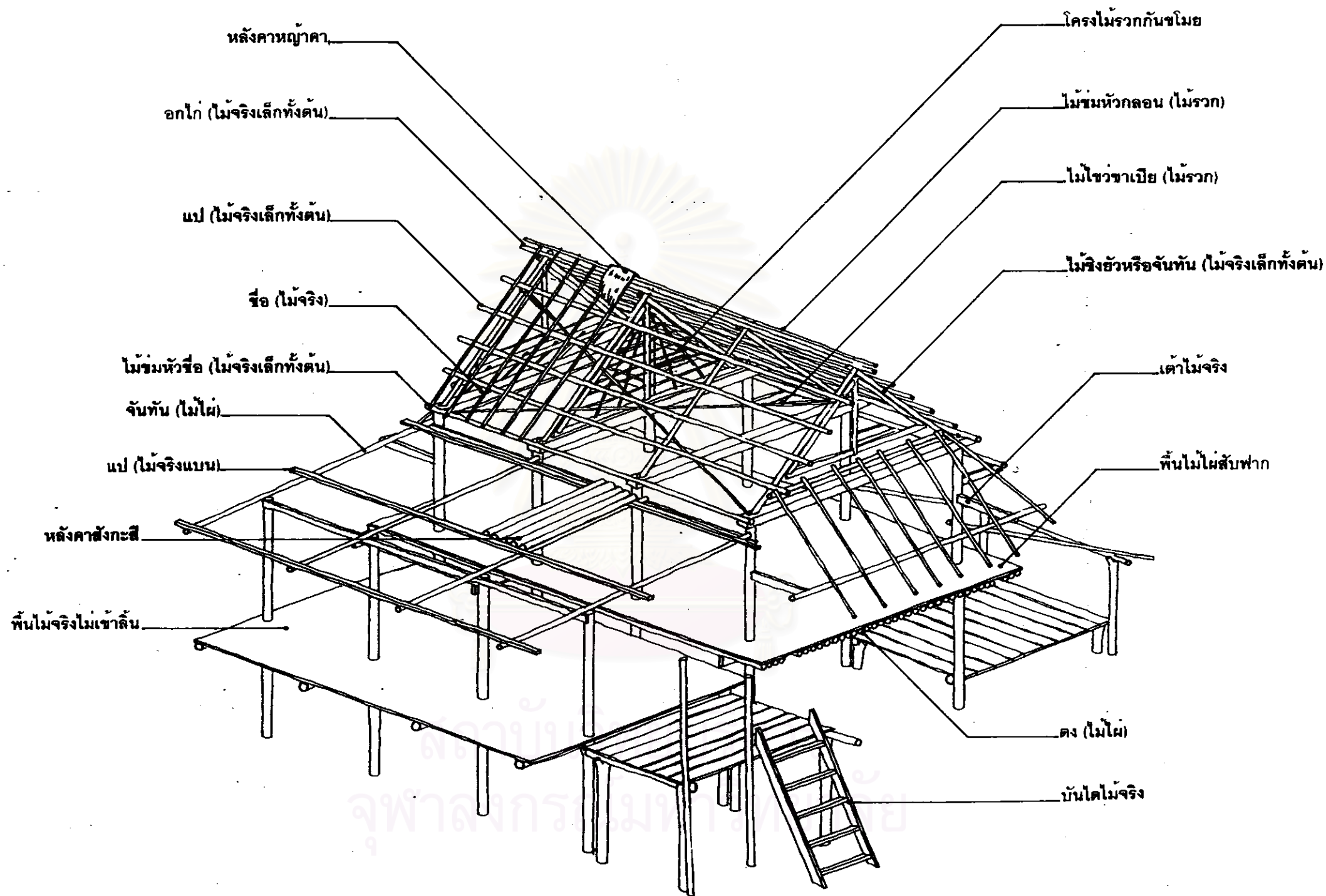
โครงสร้างเรือนนางอัด แก้วผลึก
