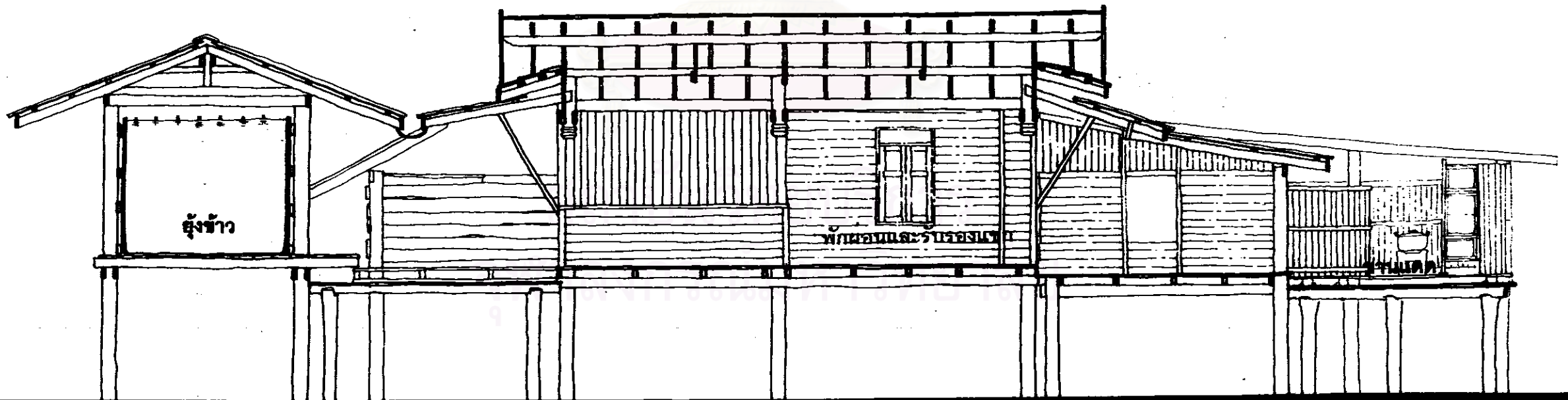
รูปตัด ข.
