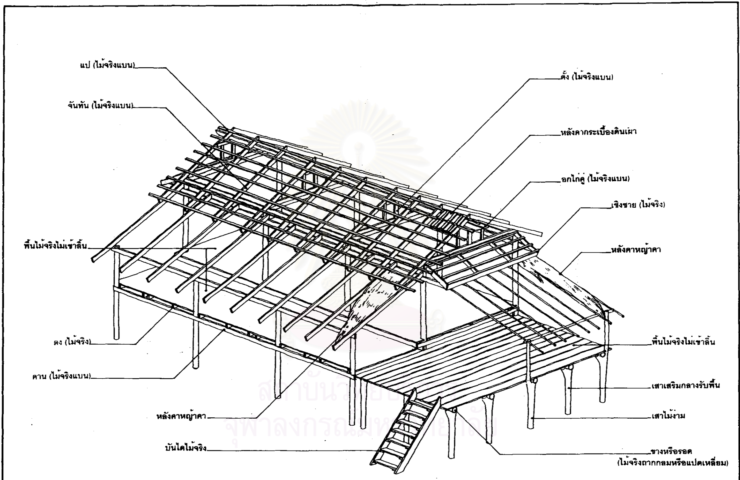
โครงสร้างเรือนนางพลอย ขึ้นถั่ว
