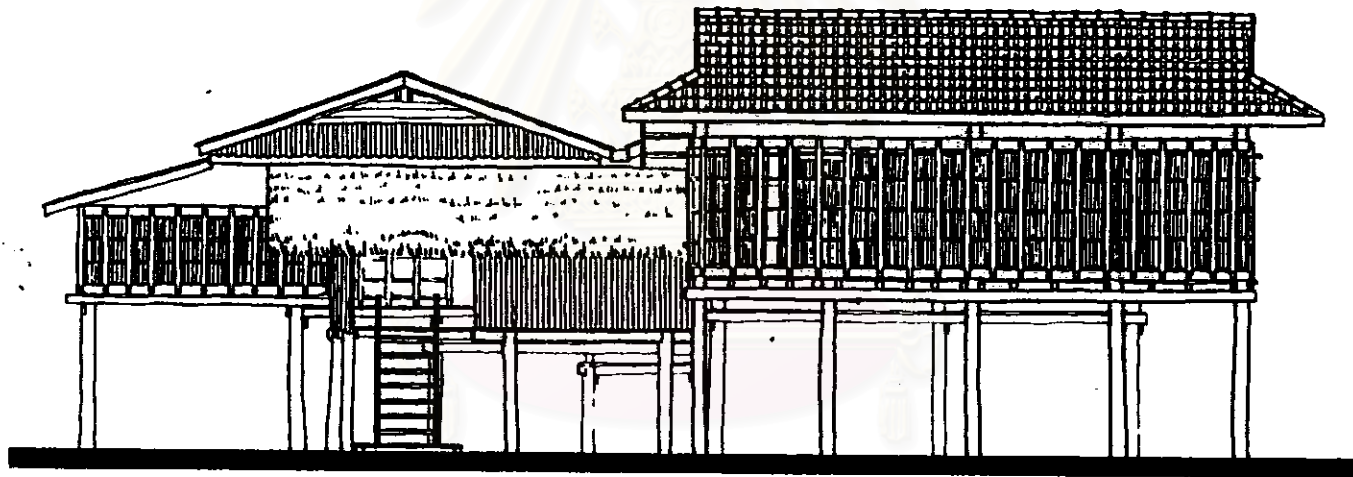
สถาบันวิทยบริการ จุฬาลงกรณ์มหาวิทยาลัย รูปด้านหน้า 0 1 3 5
