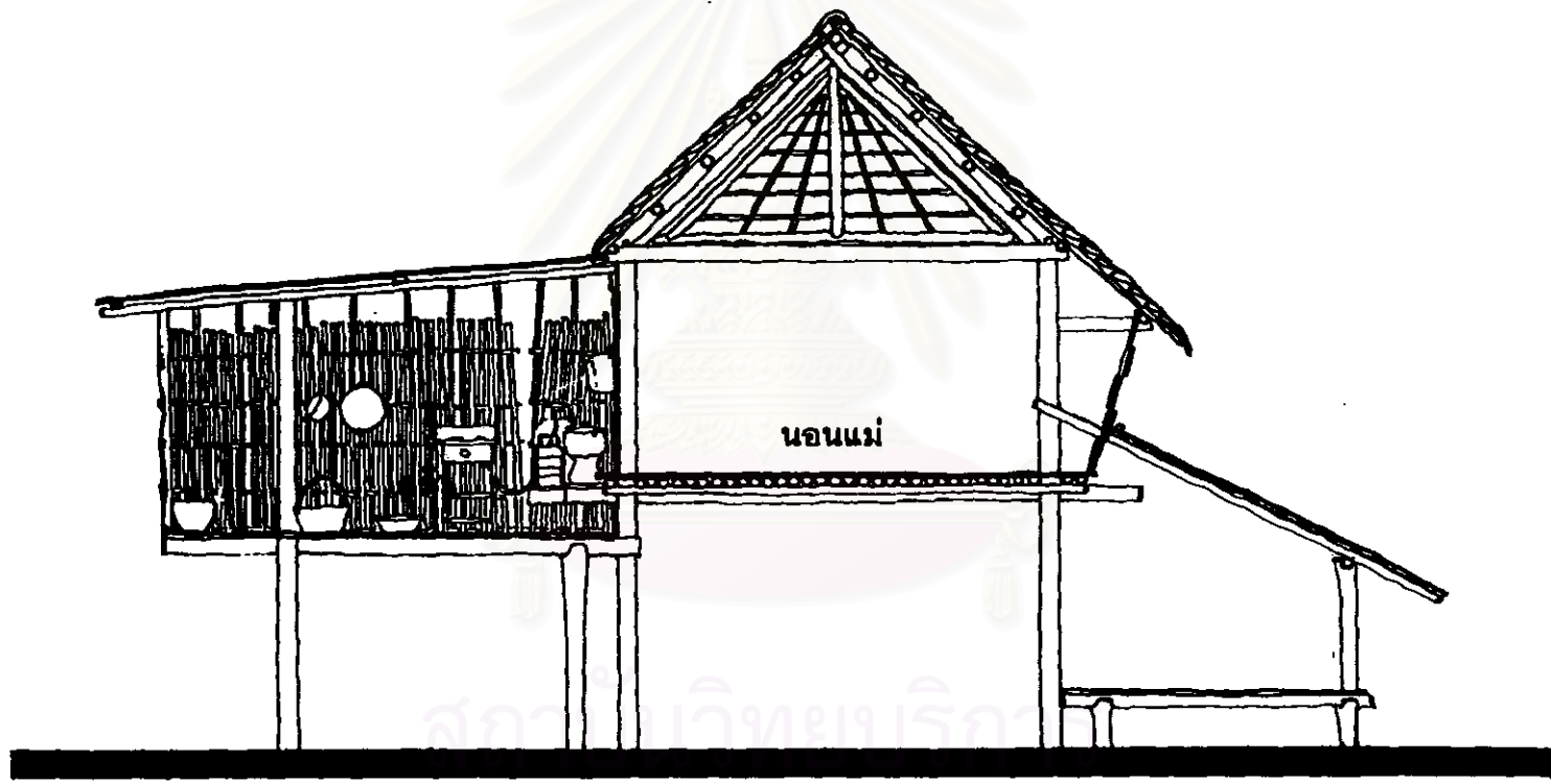
รูปตัด ก.
