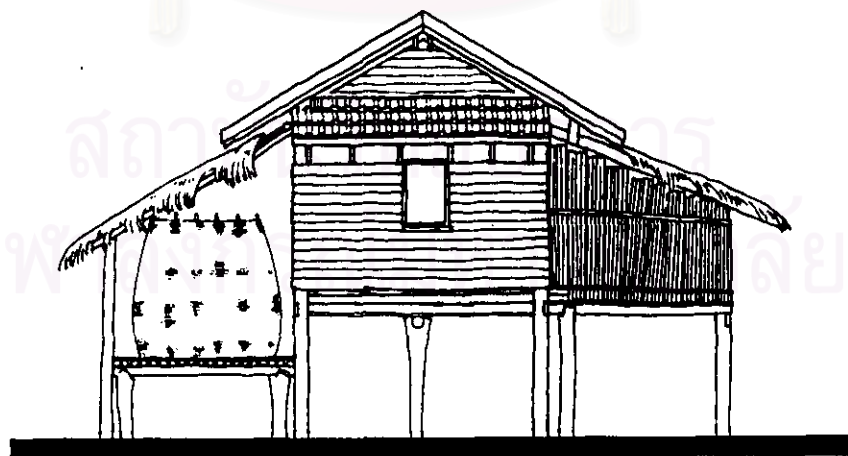
รูปด้านหลัง
