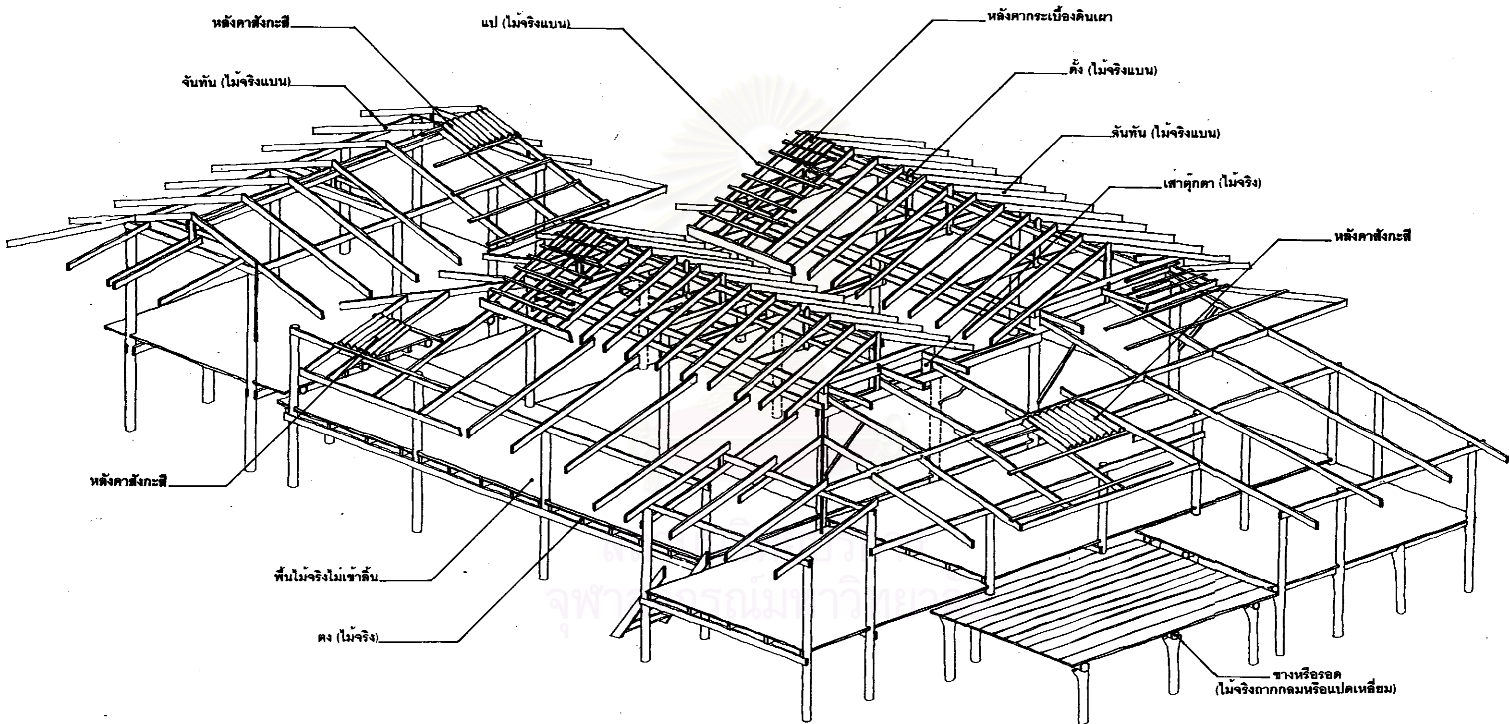
โครงสร้างเรือนนายควง พันธุ์เชื้อ
