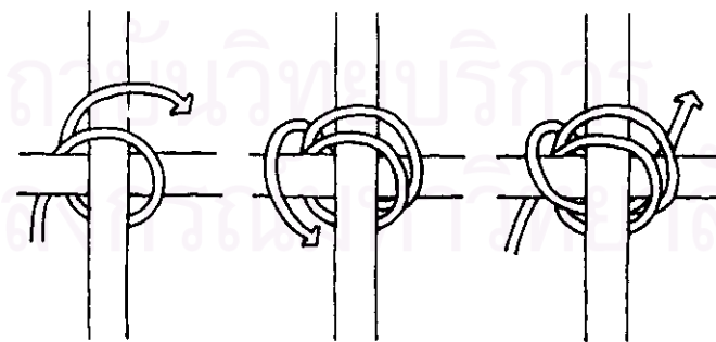
วิธีมัดแบบกำวาง
